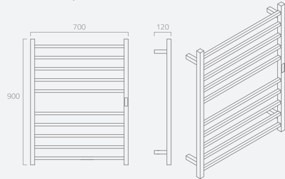
FLAT SQ10
